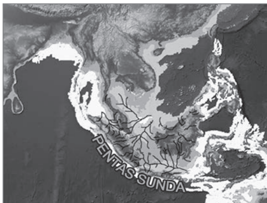
Rupa bentuk Asia Tenggara sebelum Zaman Holosen
