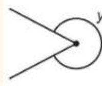
Sudut refleks Reflex angle 180^\circ < y < 360^\circ
